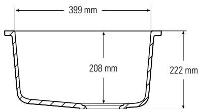
Querschnitt Seitenansicht
