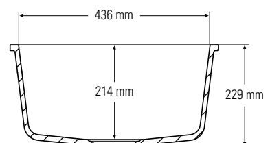
Querschnitt Seitenansicht
