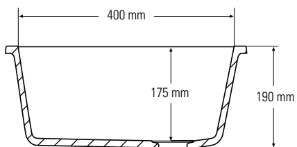
Querschnitt Seitenansicht
