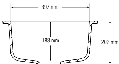
Querschnitt Seitenansicht
