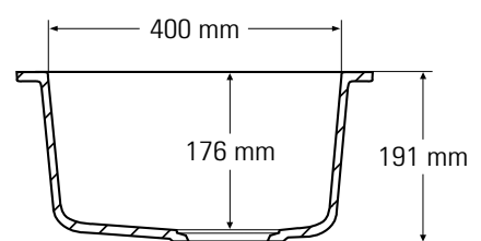
Querschnitt Seitenansicht
