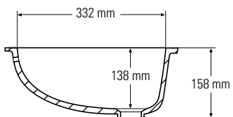
Querschnitt Seitenansicht
