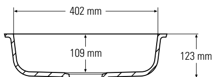
Querschnitt Seitenansicht
