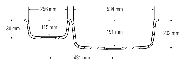
Querschnitt Seitenansicht
