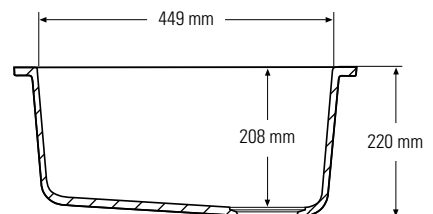
Querschnitt Seitenansicht
