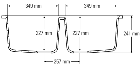
Querschnitt Seitenansicht
