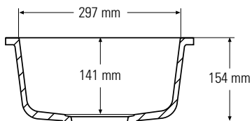
Querschnitt Seitenansicht
