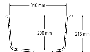
Querschnitt Seitenansicht
