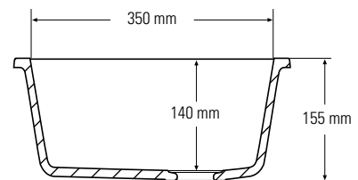
Querschnitt Seitenansicht
