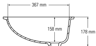
Querschnitt Seitenansicht
